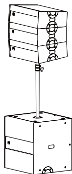
垂直阵列支撑
